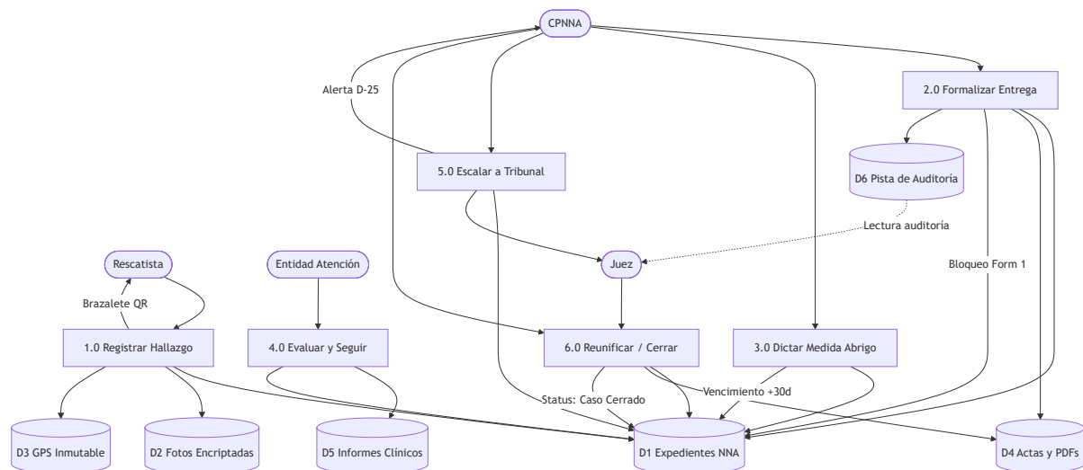
DFD Nivel 1 – Procesos principales y almacenes de datos
