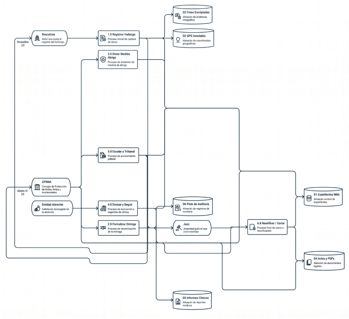
DFD Nivel 1 – Procesos principales y almacenes de datos
